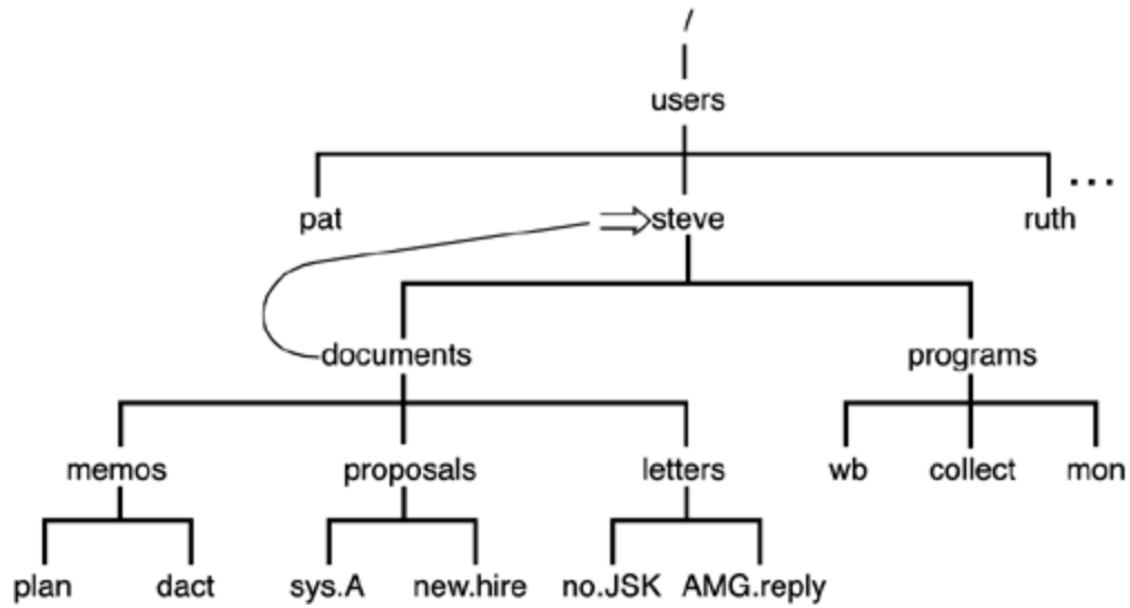
Figure 2.6. cd ..
